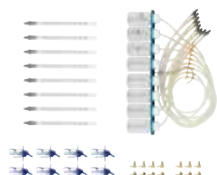
#818009 Common-Rail-Injektoren-Prüfsatz für 8 Zylinder
