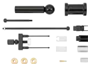
#805012 Injektor Ausziehwerkzeugsatz Zur fachgerechten Demontage und Montage von Injektoren/ Einspritzventilen sowie der Pumpe-Düse Einheit.
