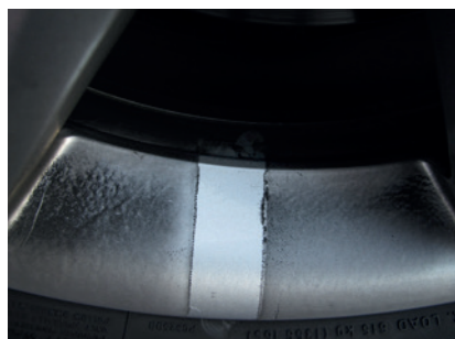
Vergleich: Felge nach Bremsungen mit Standardbelag
